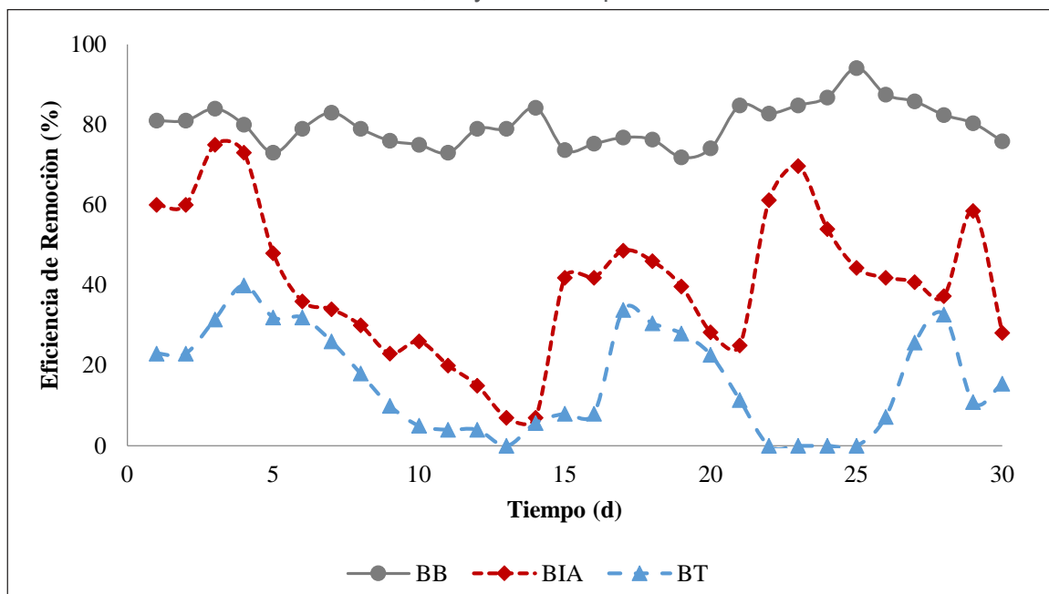
Figura 4. Remoción de nitrato en agua subterránea. Se realizaron cambios de la BIA los días 10, 17, 22 y 28 del experimento
